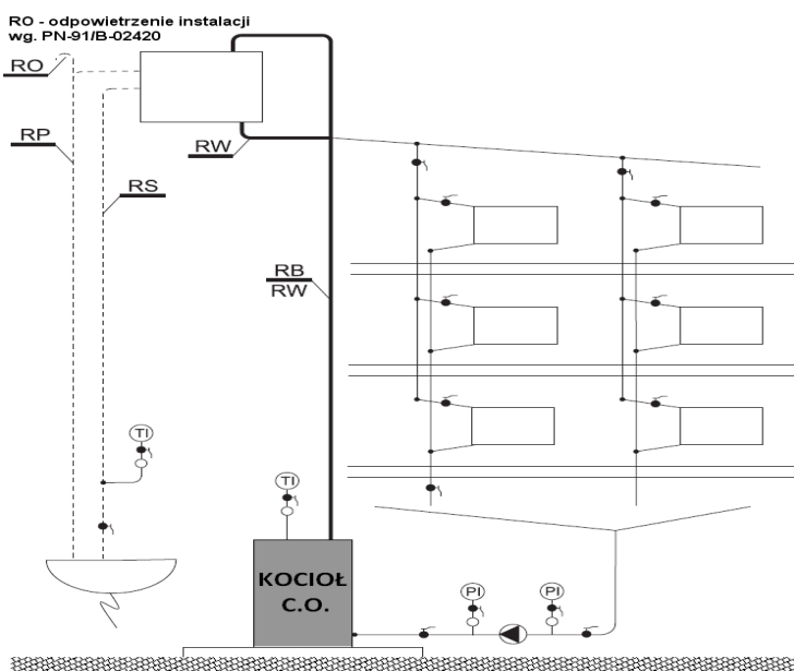
Rys. 6. Przykładowy schemat zabezpieczenia instalacji ogrzewania wodnego wyposażonej w jeden kocioł, pompa zamontowana na powrocie (wg PN-91/B-02413).
